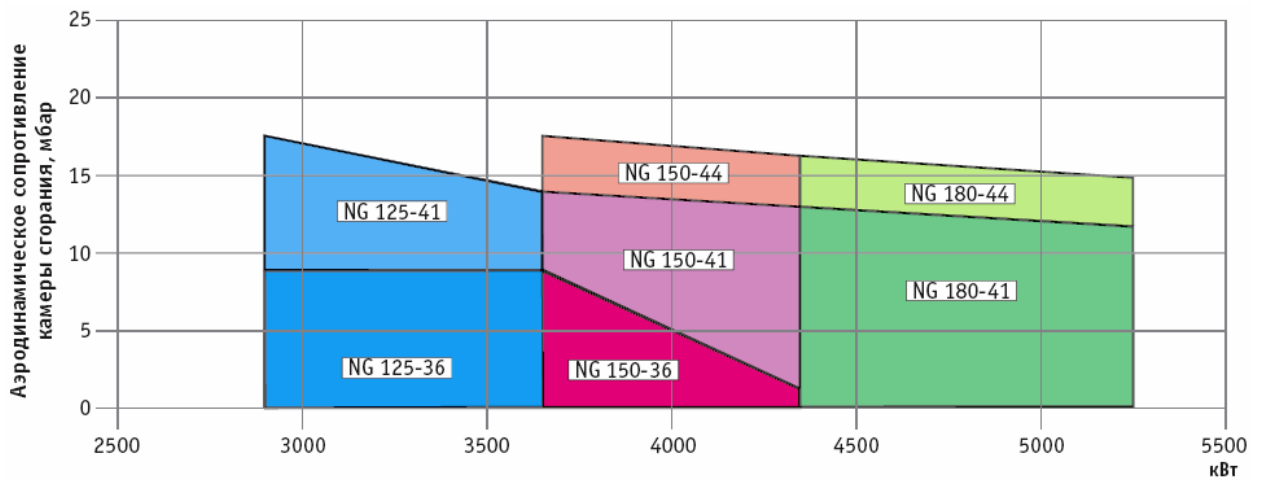
График составлен для природного газа с теплотворной способностью 38.56 МДж/м 3
